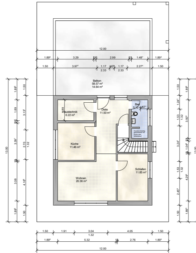
Obergeschoss M 1:200
