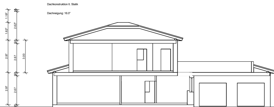
Schnitt A
