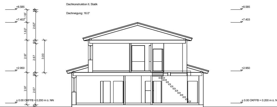
Schnitt B
