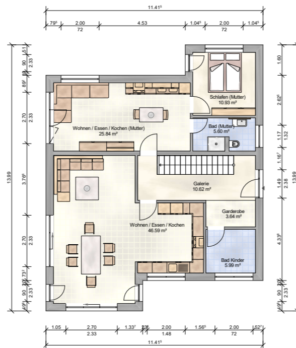
Erdgeschoss M 1:200
