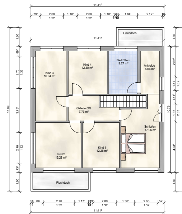
Obergeschoss M 1:200
