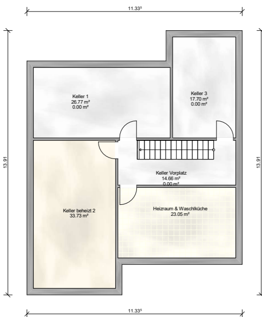
Kellergeschoss M 1:200
